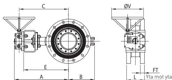
EN 1092-1 PN 16 - Utf. B
