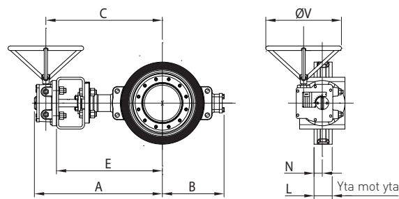
EN 1092-1 PN 25 - Utf. B
