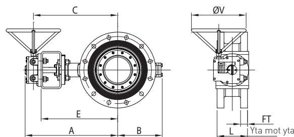
EN 1092-1 PN 40 - Utf. C
