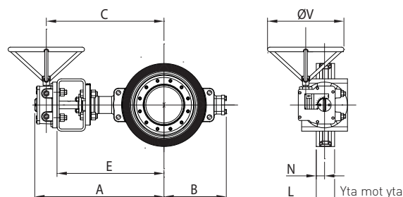
EN 1092-1 PN 25 - Utf. B
