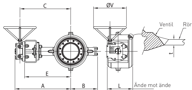
EN 12516-1 PN 40 - Utf. C
