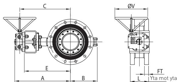
EN 1092-1 PN 25 - Utf. B
