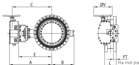
ASME B16.47 Klass 600 Serie A
