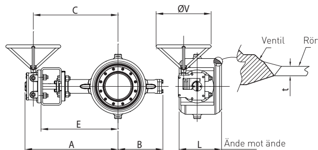
EN 12516 PN 10 - 16 - 25 - Utf. B
