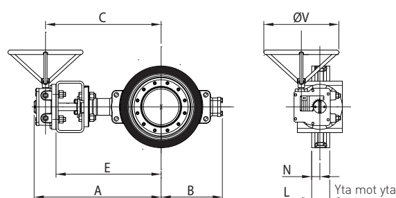
EN 1092-1 PN 10 / PN 16 - Utf. B
