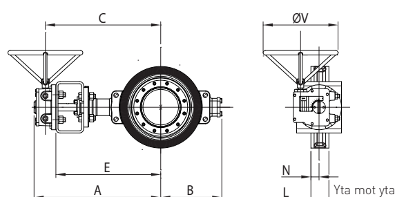
EN 1092-1 PN 40 - Utf. C
