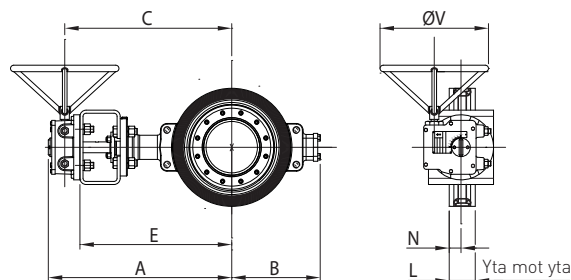
EN 1092-1 PN 40 - Utf. C
