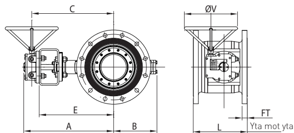
ASME B16.47 Klass 150 Serie A
