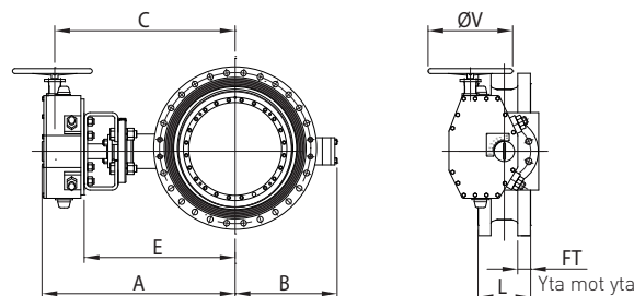
ASME B16.47 Klass 900 Serie A
